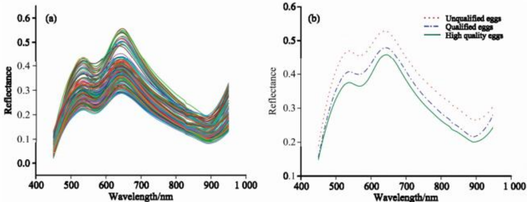
图 3 样本原始光谱(a), 样本平均光谱(b) Fig. 3 Original (a) and mean (b) spectra of egg samples
