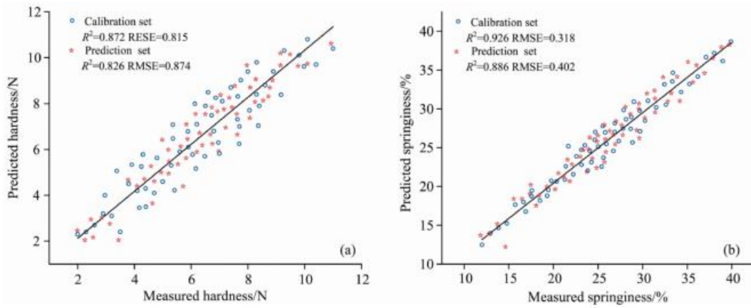
图 8 质构硬度验证散点图 (a), 弹性验证散点图 (b)
