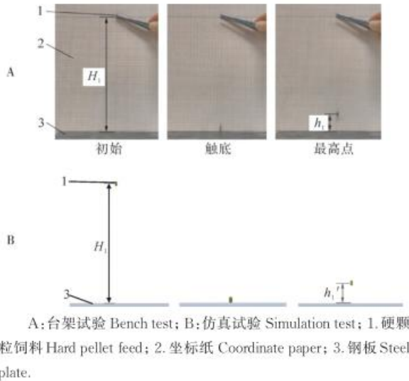
图3 碰撞恢复系数标定试验
