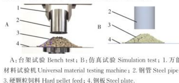
图6 堆积角试验
