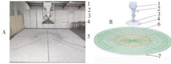
图9 硬颗粒饲料抛撒试验 A: 台架试验 Bench test; B: 仿真试验 Simulation test; 1. 料箱 Hopper; 2. 下料辊 Blanking roller; 3. 离心转盘 Centrifugal turntable; 4. 圆台挡板 Frustum baffle; 5. 收集区域 Collection area; 6. 饲料质量检测区域 Feed quality inspection area; 7. 落料圆板 Circular plate for collecting feed.
