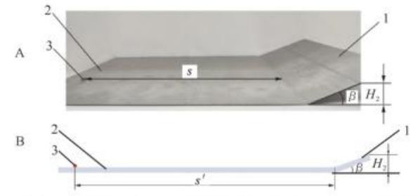
A: 台架试验 Bench test; B: 仿真试验 Simulation test; 1. 倾斜钢板 Inclined steel plate; 2. 平置钢板 Flat steel plate; 3. 硬颗粒饲料 Hard pellet feed.
