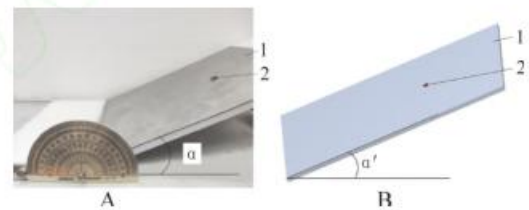
图4 静摩擦因数标定试验
